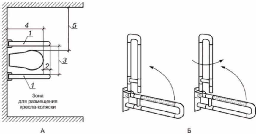
Расположение поручней возле унитаза принято согласно рис.19 ГОСТ 51261-2022.
