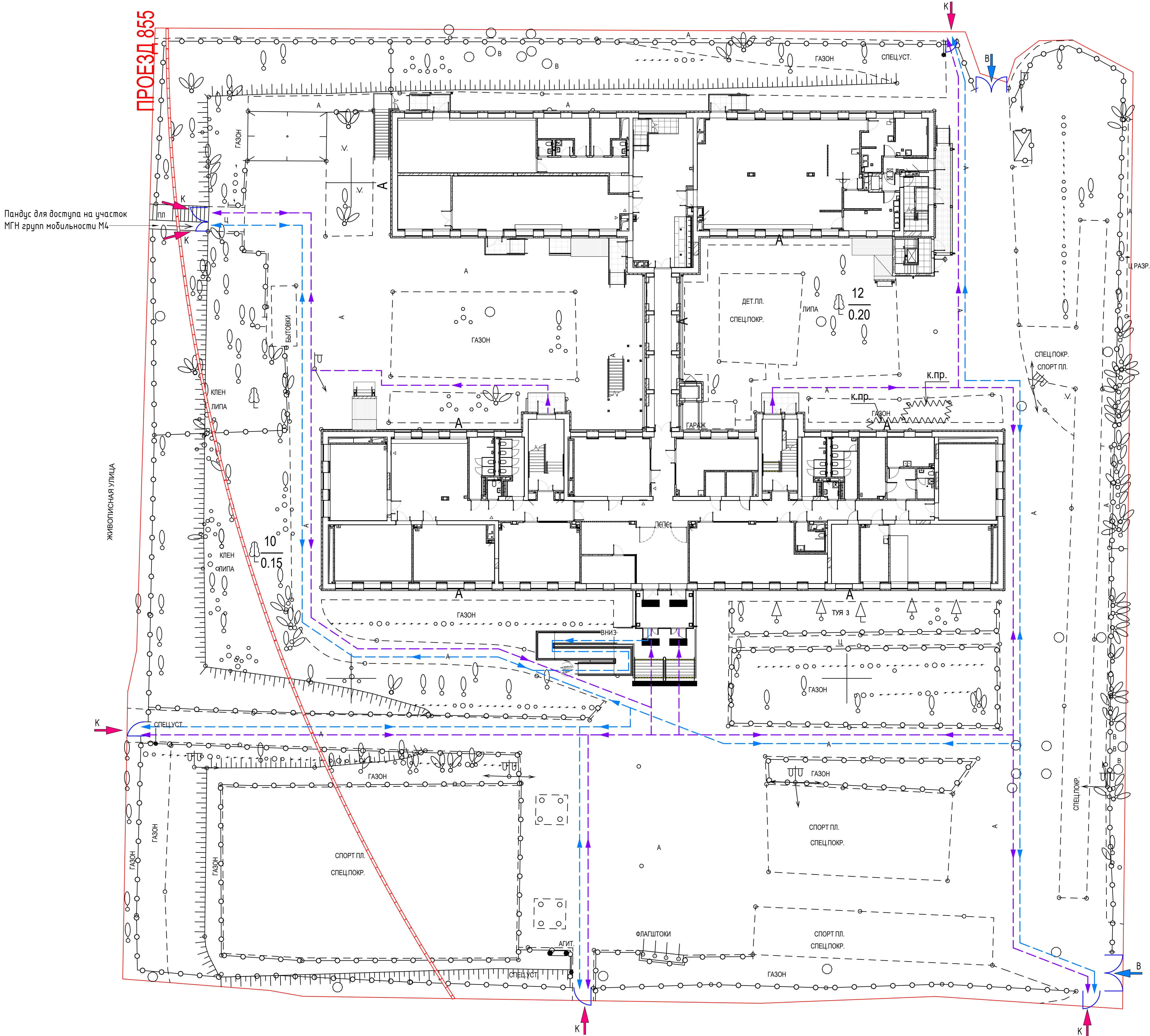
Схема организации земельного участка с указанием путей перемещения маломобильных групп населения М1-М3, М4 М 1:200
