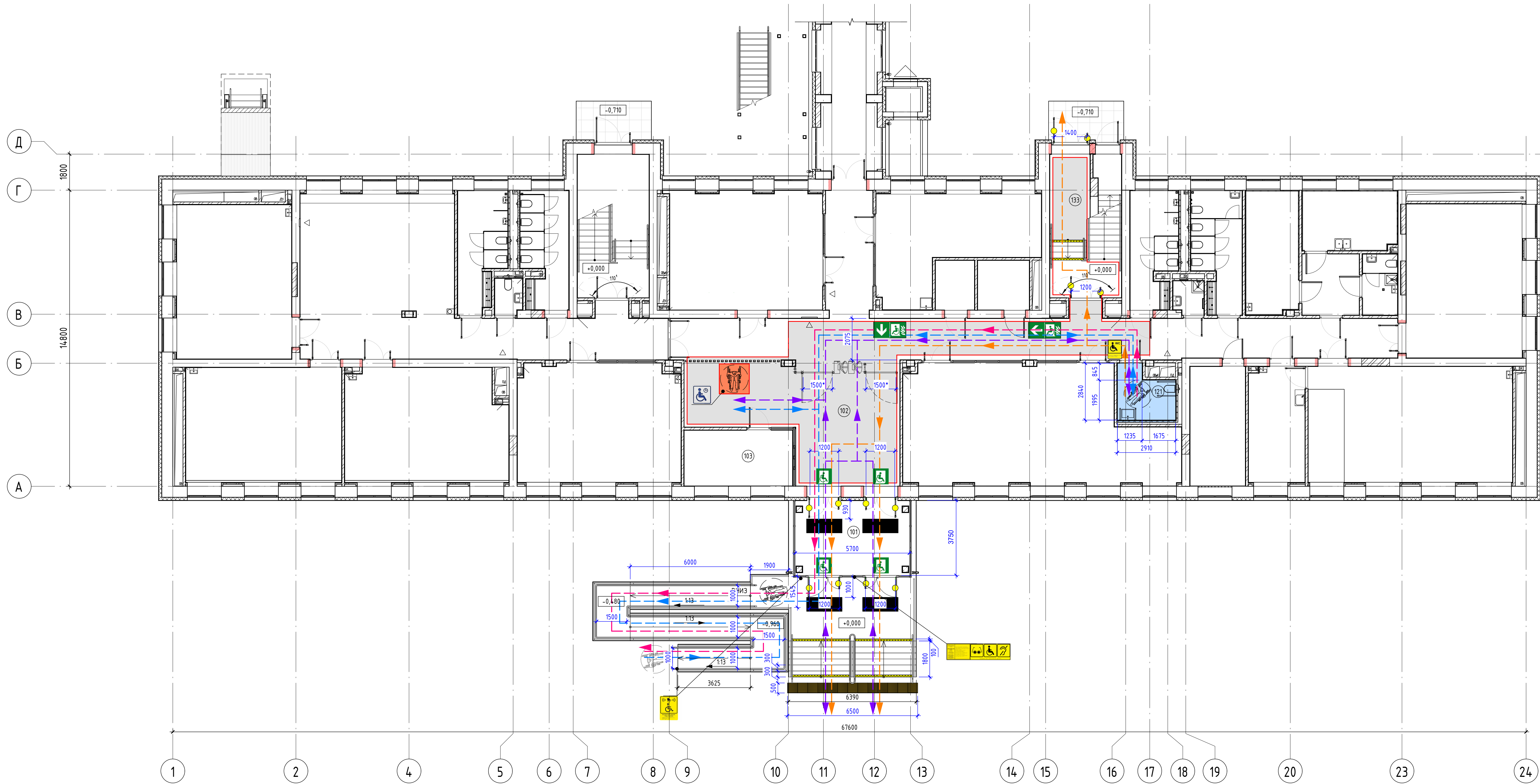
Фрагмент плана 1 этажа со схемой движения МГН
